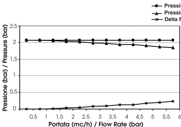
Cartuccia 20" FA-BIG 5 µ con filtro Aqua Big attacchi 1" / 20" FA-BIG 5 µ cartridge with 1" Aqua Big filter
